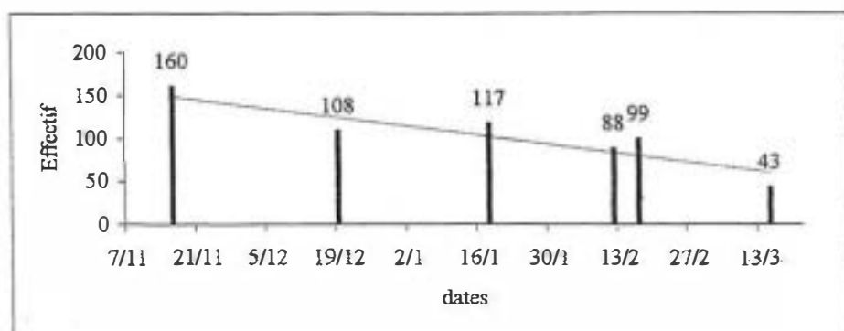
Aigrette garzette au dortoir de Kerner / Riantec (Morbihan) ; hiver 2001-2002
