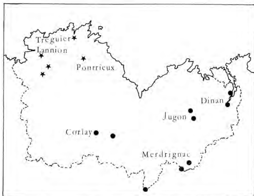
Les captures de Rats musqués dans les Côtes-du-Nord en 1958-59 (cercles) et en 1962-63 (étoiles)
