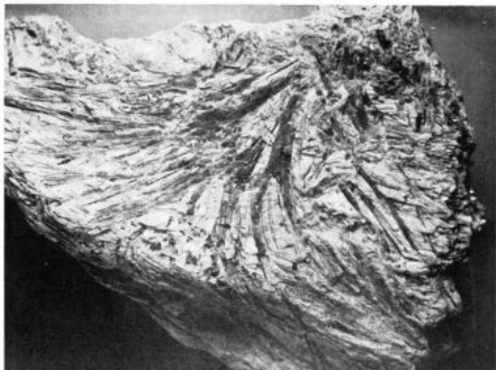
Fig. 31. — Actinotite massive avec cristaux bien individualisés ( \times 3/2 ). Falaise Ouest du Sémaphore.
