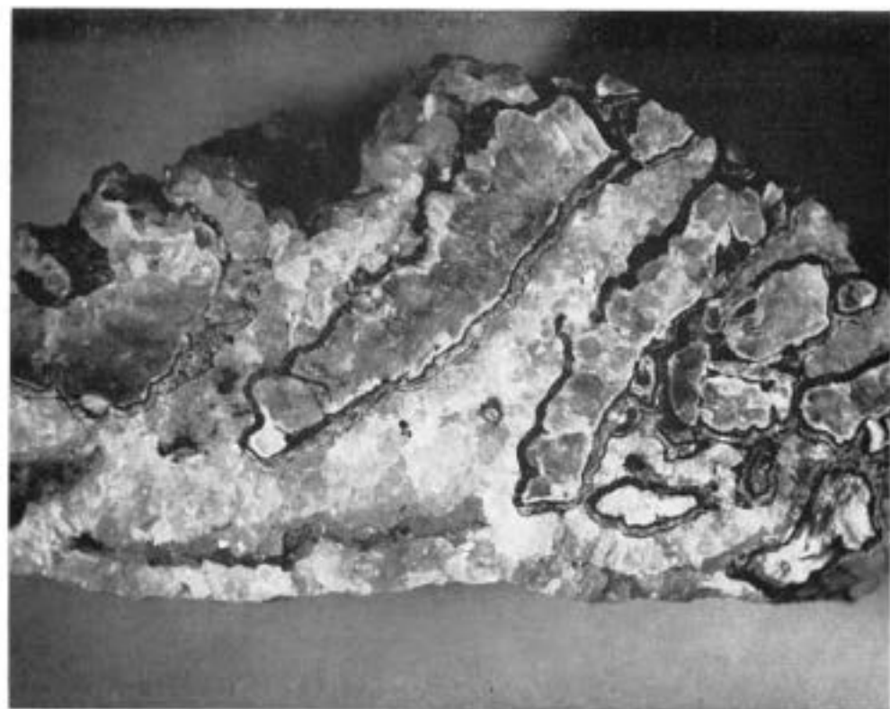
Fig. 18. — Blende et galène (noir) dans quartz (blanc) ( \times 1 ). Halde de Poullaba, près du Huelgoat (Finistère).
