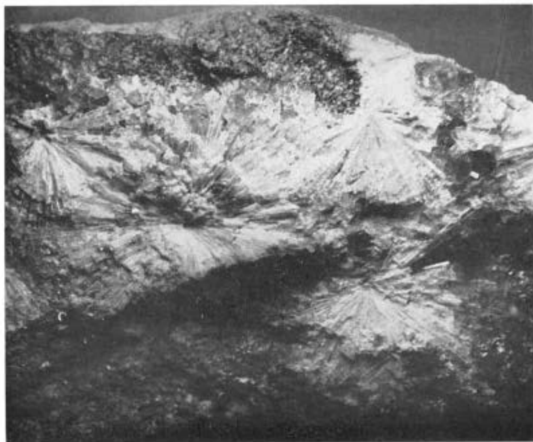
Fig. 12. — Rosaces de beryl sur le granite ( \times 3/2 ). Menez-Gouaillon en Coray (Finistère).
