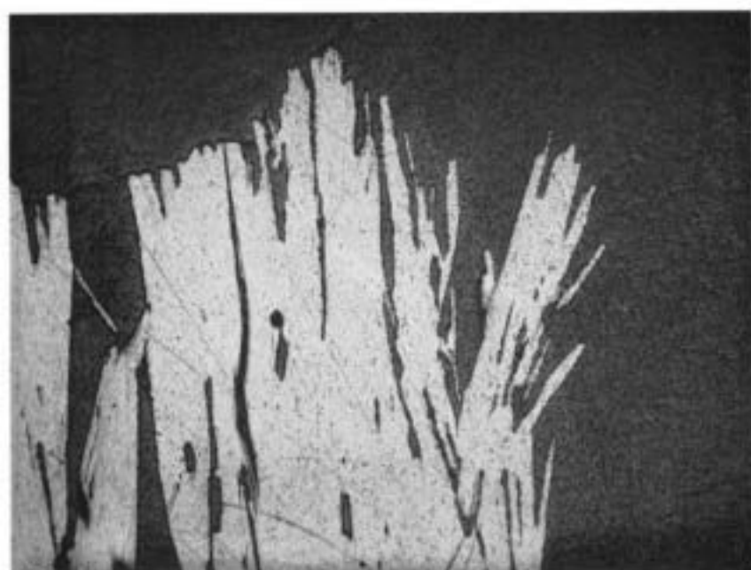
Fig. 15. — Molybdénite dans feldspath. Section polie observée au microscope métallographique (L.N. \times 45 ). Ploumanach (Côtes-du-Nord).
