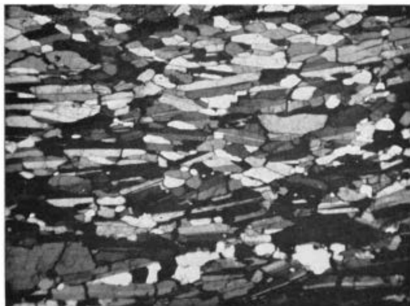
Fig. 9. — Aprite à albite (albiteite), observée au microscope polarisant (L.P. \times 45 ).
