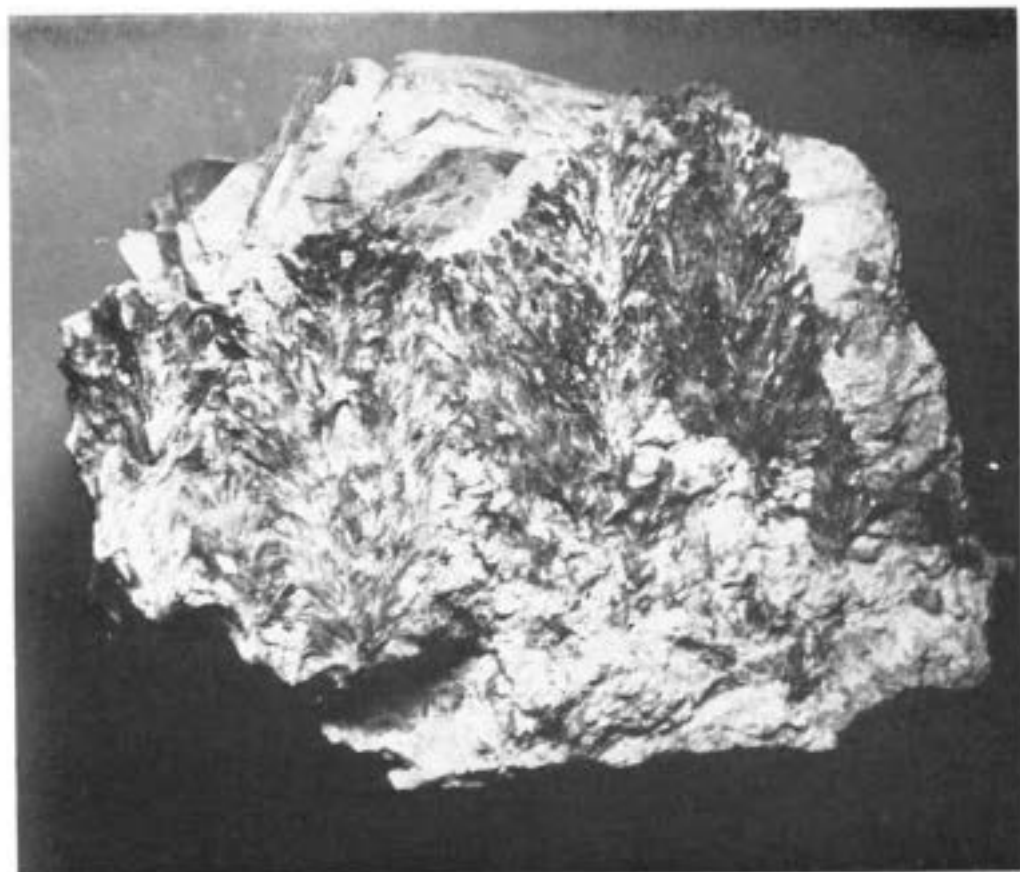
Fig. 10. — Pegmatite à mica palmé ( \times 4/3 ). Menez-Gouaillon en Coray (Finistère).
