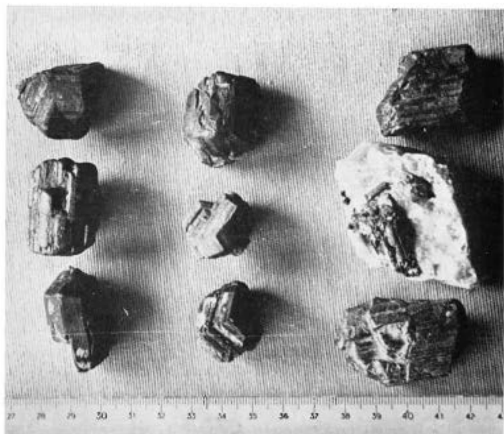
Fig. 6. — Rutile de Kerleven
