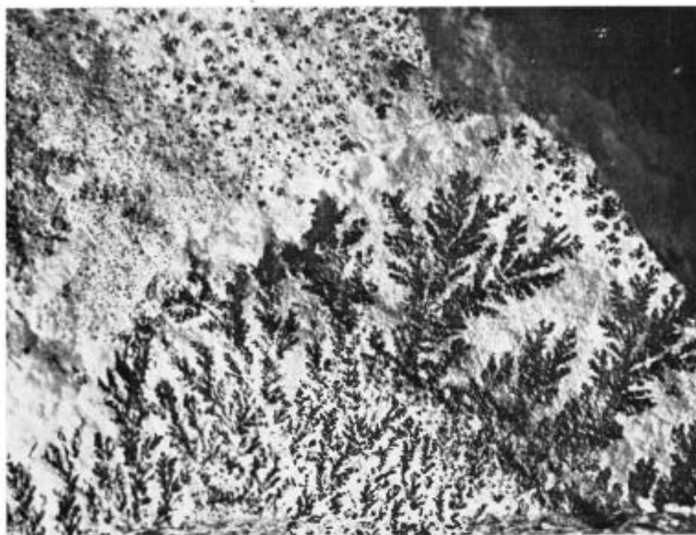
Fig. 26. — Carrière du bois de Lemezec, au Sud de Scrignoac. Dendrites de manganèse dans les fissures de l'aplite.
