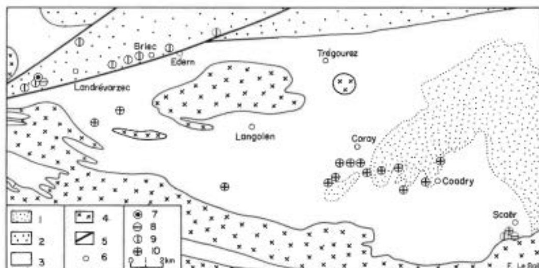
Fig. 46. — 1 : Placage tertiaire — 2 : Paléozoïque — 3 : Briovérien — 4 : Granite — 5 : Faille — 6 : Localité — 7 : Grenat — 8 : Andalousite — 9 : Disthène — 10 : Staurotide.
